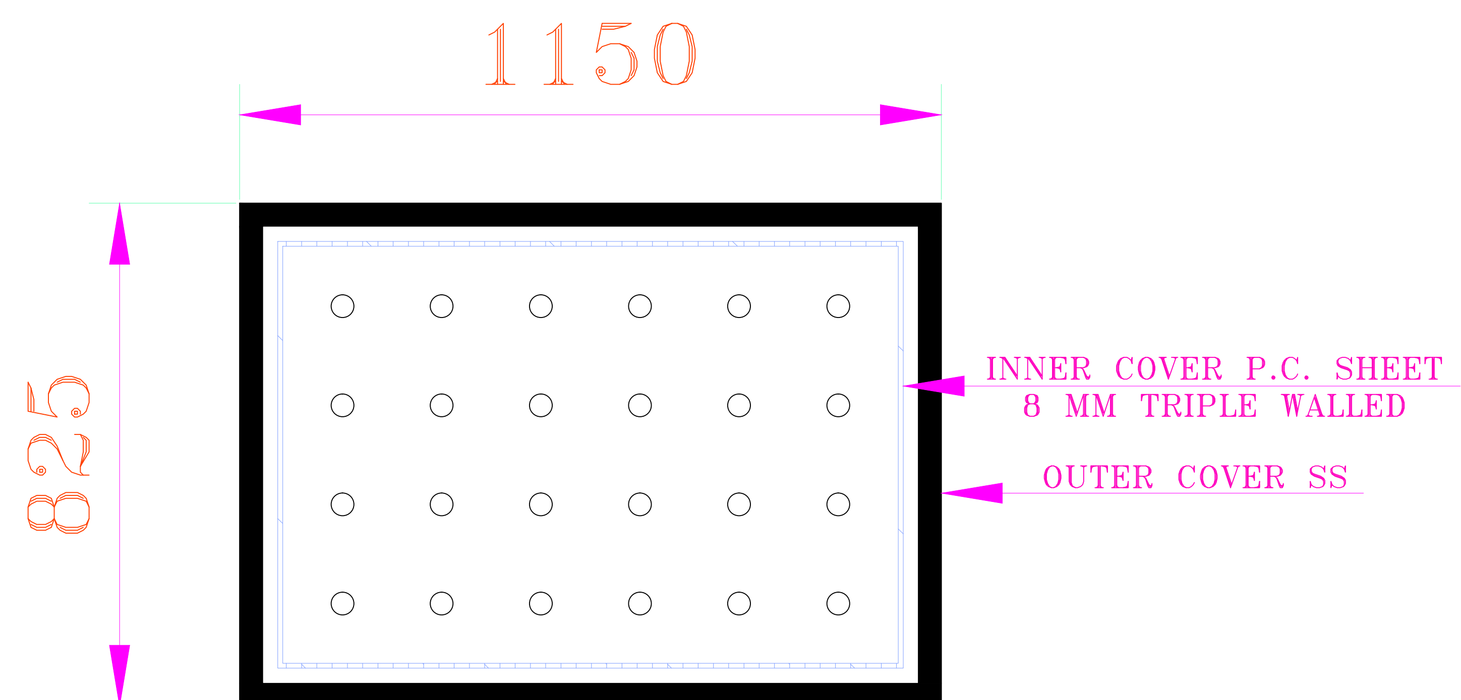
PLAN MINI AEROPONIC BOX
